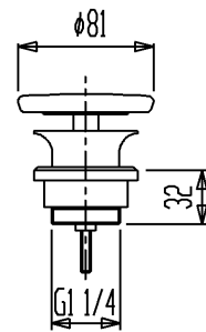
排水目皿付 (尺度 1:5)
