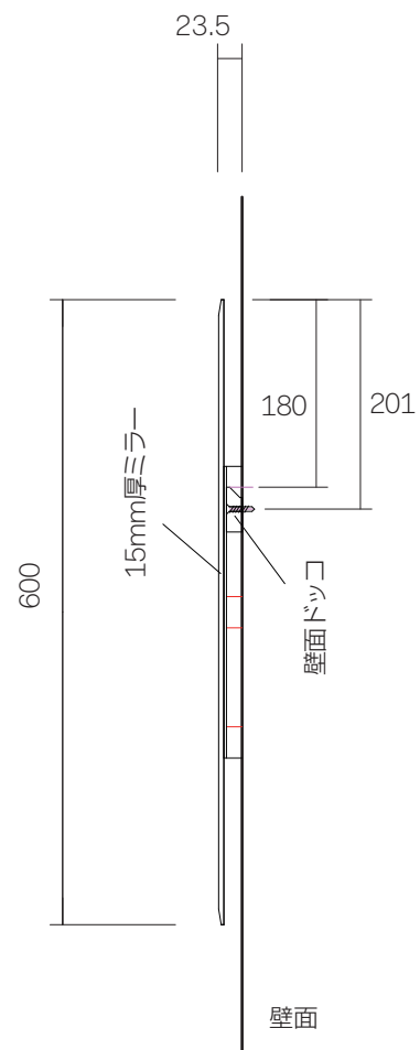
壁面取付図
