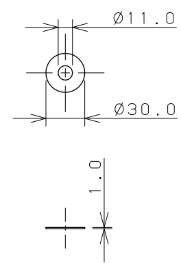
スリップワッシャ (X2)
