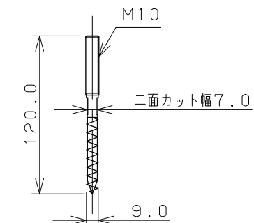
ハンガーボルト (X2)
