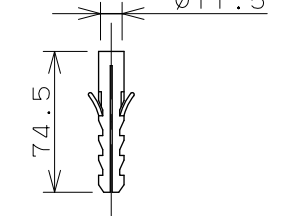
アンカープラグ (X2)
