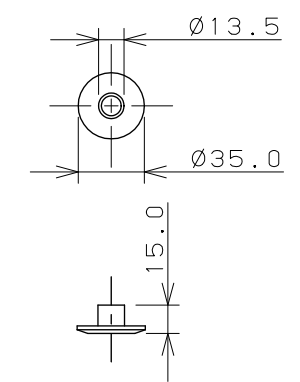
スペーサー (X2)
