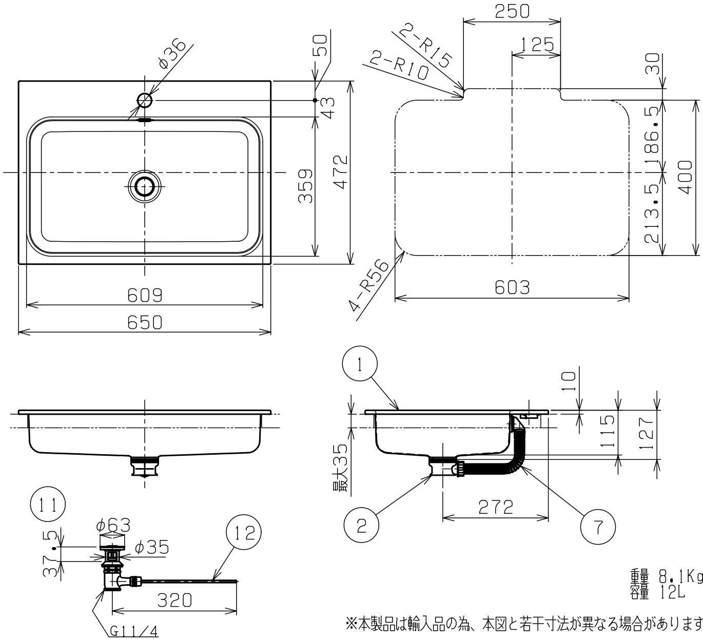
カウンター切込寸法図
