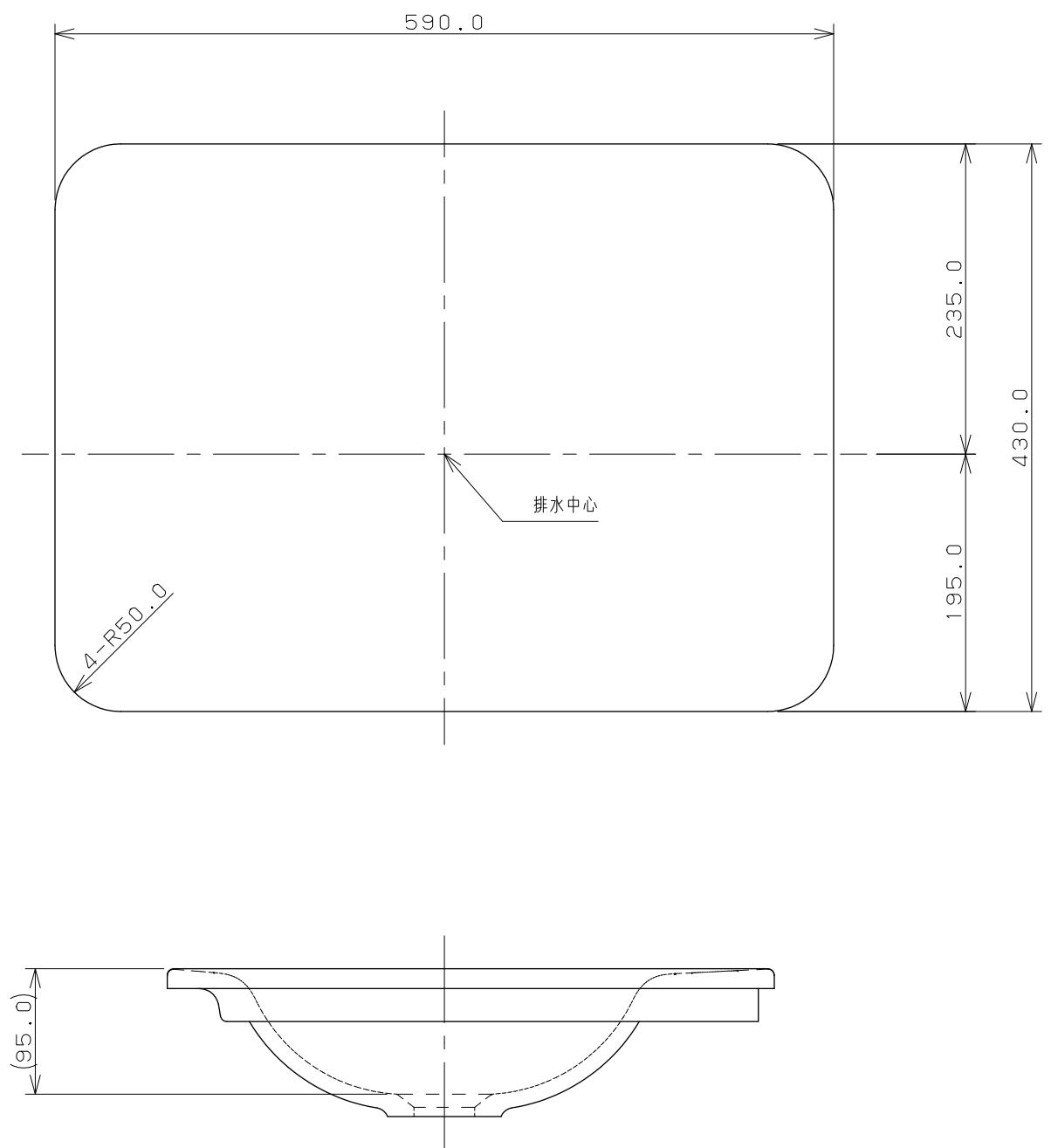
カウンター切込寸法
