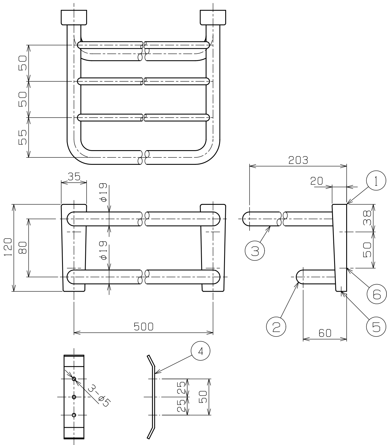
標準パイプ寸法 L-500m/m
