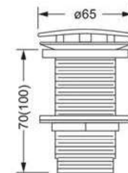
JORGER排水栓本体図
