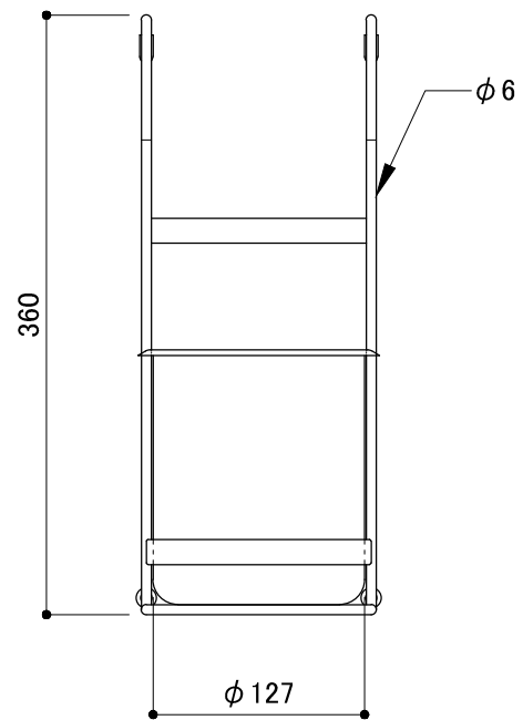
レーリングシステム LINERO 調理用具ホルダー 大 Art.No. 521.19.311
