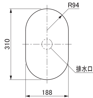
カウンター切込寸法
