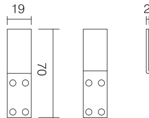
取り付け金具形状
