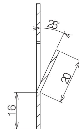
断面図 A-A
