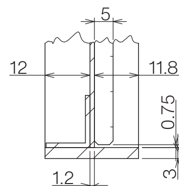
詳細図 B
