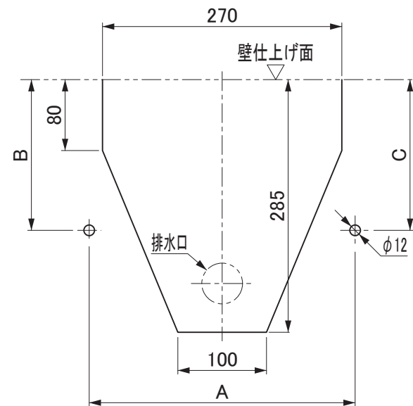
カウンター切り込み寸法
