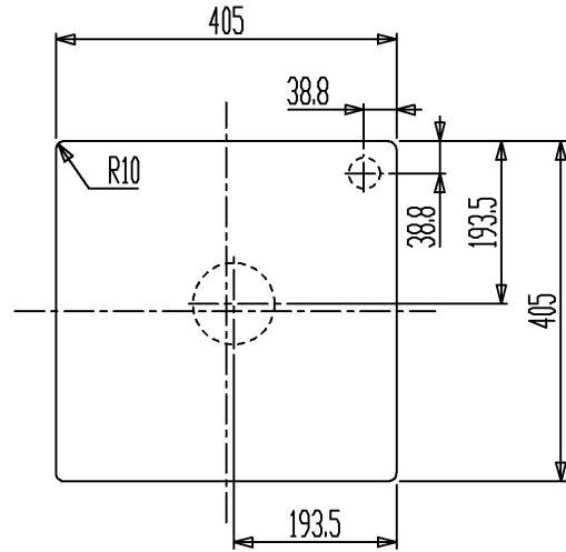
カウンター切込寸法
