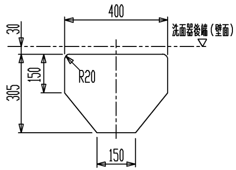
カウンター切込寸法 ※カウンターを設ける場合
