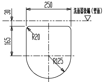
カウンター切込寸法 ※カウンターを設ける場合
