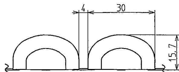
B部詳細図 (1:1)
