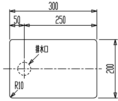
カウンター切込寸法
