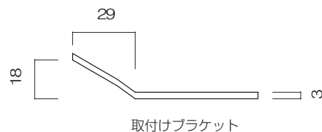
取付けブラケット
