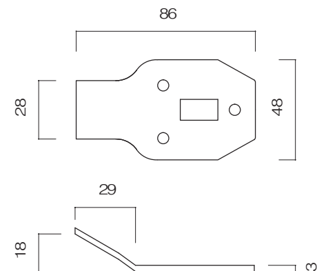
取付けブラケット 単位:mm
