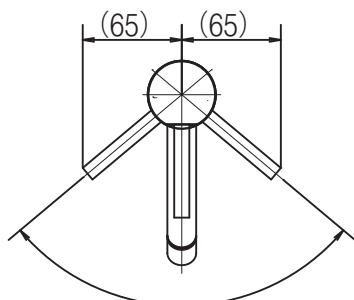
レバー 約100°
