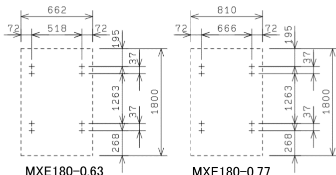
取付け金具ビス穴位置
