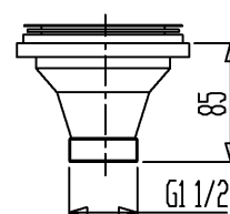
排水金具付
