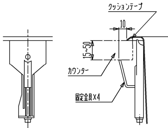
固定部詳細 1:3
