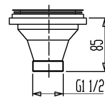
排水目皿付
