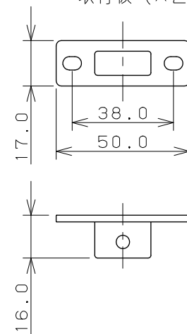
取付板 (X2)
