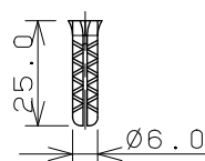
プラグ (X4)
