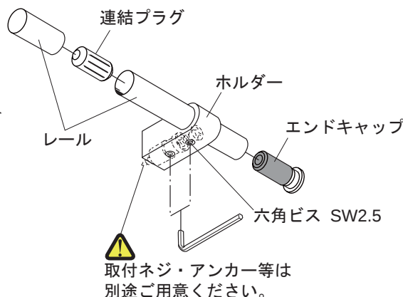
エンドキャップ φ16mmレール用
