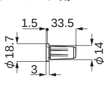
連結プラグ φ16mmレール用
