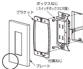
コンセント
