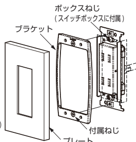
コンセント
