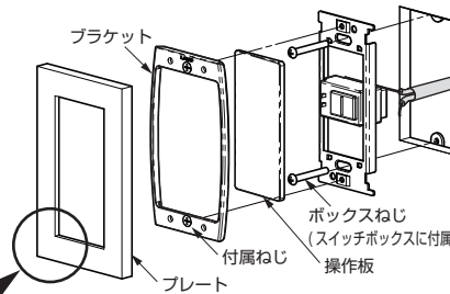
スイッチ
