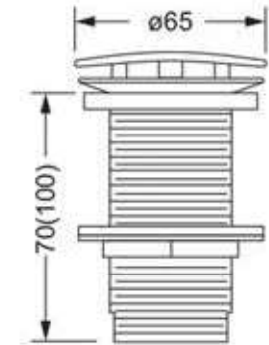
JORGER排水栓本体図
