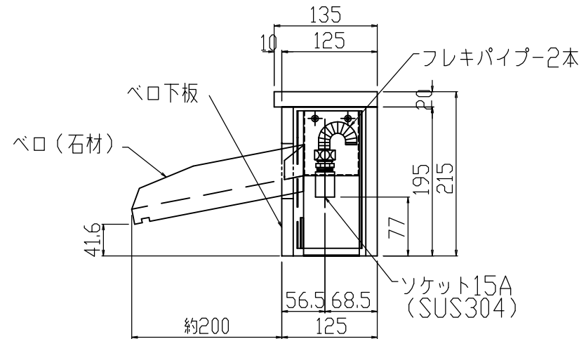
断面
