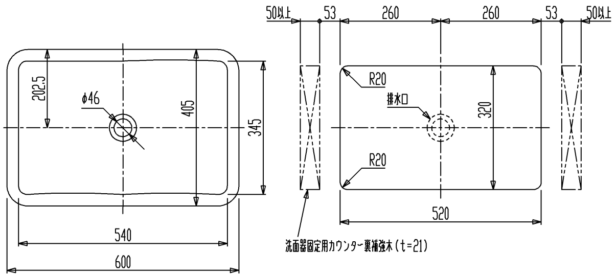
カウンター切込寸法
